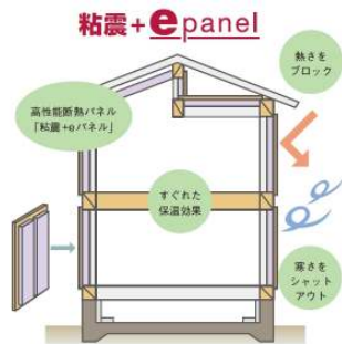
《図2:オリジナル高性能パネル「粘震+eパネル」》
